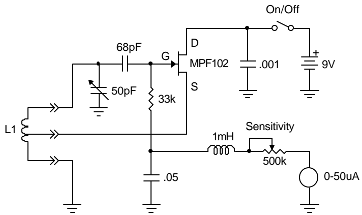
Dip Meter
